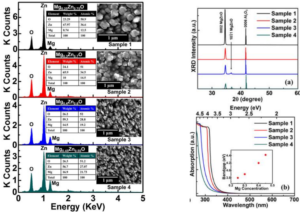
左图为 MgZnO 薄膜的组成和形貌。分别为样品 1 (Mg0.25Zn0.75O)，样品 2 (Mg0.3Zn0.7O)，样品 3 (Mg0.4Zn0.6O) 和样品 4 (Mg0.45Zn0.55O)。右图为 MgZnO 薄膜的结构和带隙特性。(a) MgZnO 薄膜的 XRD 光谱 (样品 1-4)。(b) MgZnO 薄膜的室温吸收光谱 (样品 1-4)，插图显示了膜中 Mg 含量的带隙变化。
