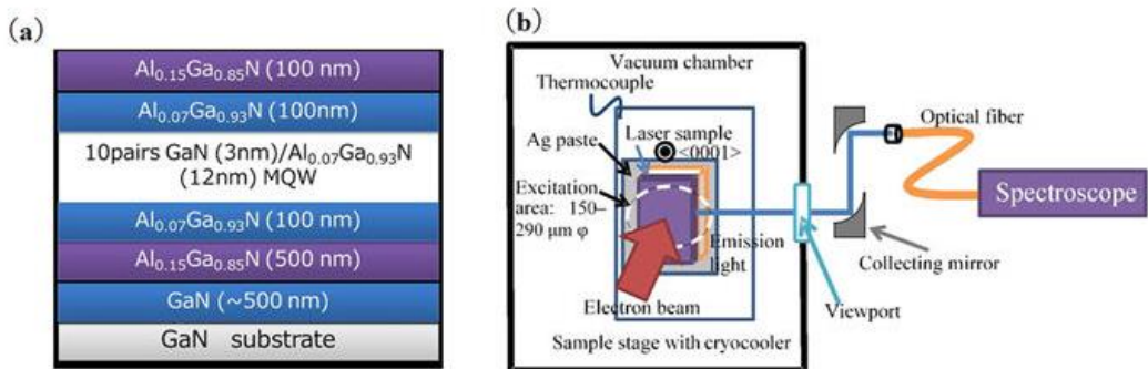
图 (a) 为激光器结构的示意图，其包括在 c 面独立的 GaN 衬底上生长的具有 GaN/AlGaN MQW 有源层分离的限制异质结构。该结构的光学约束因子约为 6%。三甲基铝、三甲基镓、三乙基镓和氨用作源气体。堆叠依次包括 500nm 厚的同质外延 GaN 层，500nm 厚的 Al 0.15 Ga 0.85 N 纳米包层，100nm 厚的 Al 0.07 Ga 0.93 N 光导层，10 对 GaN (3nm) 和 Al 0.07 Ga 0.93 N (12nm) 作为 MQW 有源层，100nm 厚的 Al 0.07 Ga 0.93 N 导光层和 100nm 厚的 Al 0.07 Ga 0.93 N 包覆层。激光腔通过 Cl 2 电感耦合等离子体蚀刻和使用四甲基氢氧化铵水溶液 (25at%) 的湿蚀刻的组合形成。激光样品的腔长度约为 50 μm。由于腔长度较短，因此无涂层。图 (b) 给出了电子束激发和测量系统的示意图。将激光样品安装在装有低温冷却器的冷却台上。使用 Ag 浆料安装样品，然后使用涡轮分子泵将室抽真空至约 1×10 -5 Pa。使用 LaB 6 电子束枪作为激发源，根据电子束的加速电压求出样品的发光。
