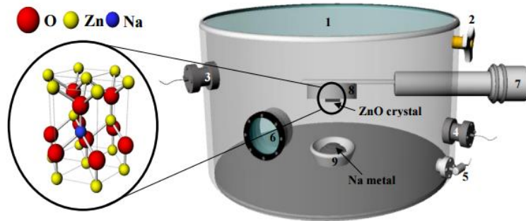
钠掺杂室示意图。(1) 室内玻璃盖 (2) 开/关闭 (3) 热通道供给 (4) 热电偶进给 (5) 泵连接器 (6) 通道 (7) 机械手 (8) 按钮加热器 (9) 氧化铝中的 Na 金属。
