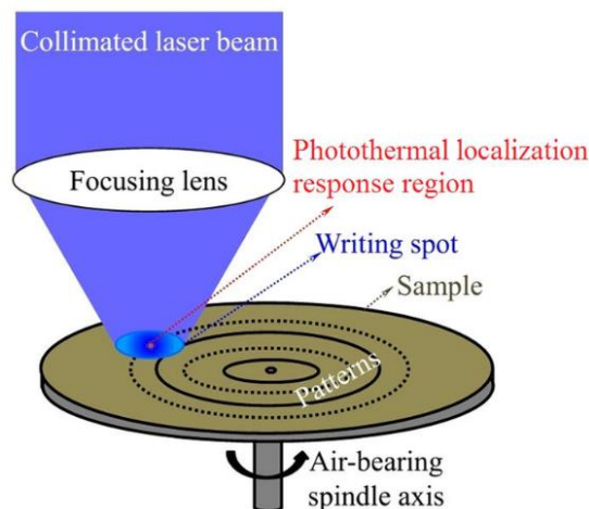
上图为在 AgInSbTe 涂层样品上的高速无掩膜纳米光刻技术的示意图，其中由于光热定
