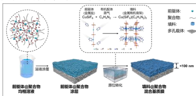
混合基质膜制备示意图
