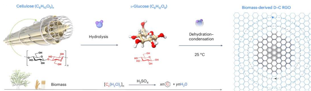
室温下生物质一步转化为还原氧化石墨烯示意图
