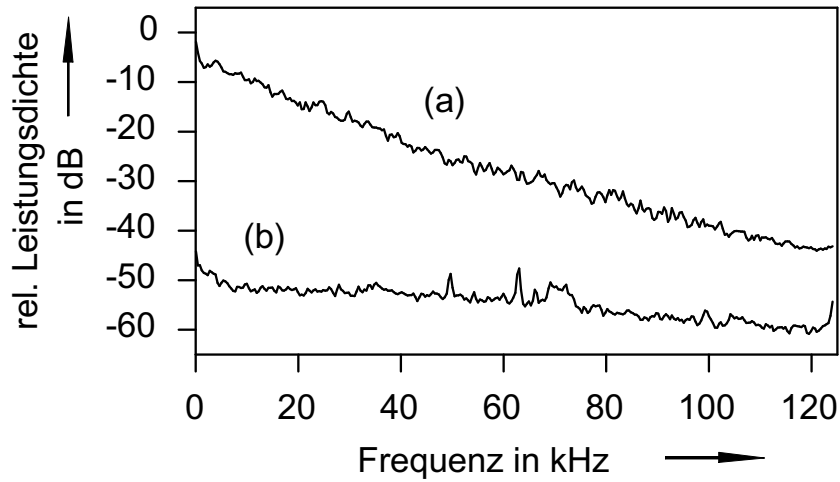
Abbildung 3.7: Spektrale Leistung der Phasenfluktuationen aufgrund von mechanischer Belastung einer Grundmodefaser. (a) unter Belastung der Faser, (b) Nullmessung der Meßelektronik zur Quantifizierung des Rauschniveaus.
