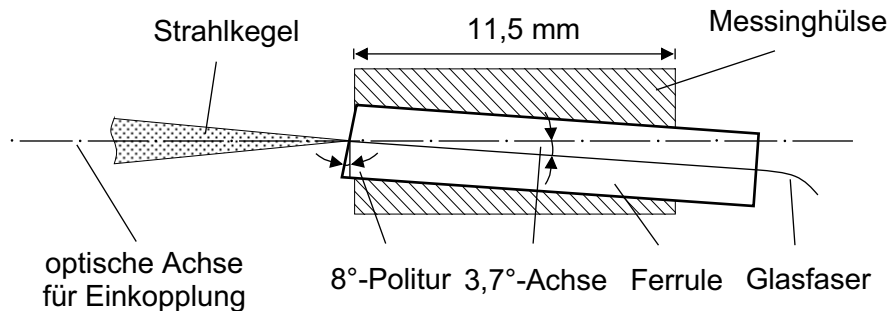
Abbildung 4.3: Montagehülse für schrägpolierte polarisationserhaltende Glasfasern. Die Bohrung unter 3,7^\circ kompensiert die Verkippung des Strahlkegels gegenüber der geometrischen Faserachse und ermöglicht damit die azimutale Justage der Fasern.
