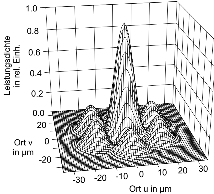
Abbildung 3.10: Berechnete Leistungsdichteverteilung für die kohärente Überlagerung von drei Einzelemittlern. Die Einzelemitter sind auf einem hexagonalen Gitter in der Ebene des Linsenarrays angeordnet.
